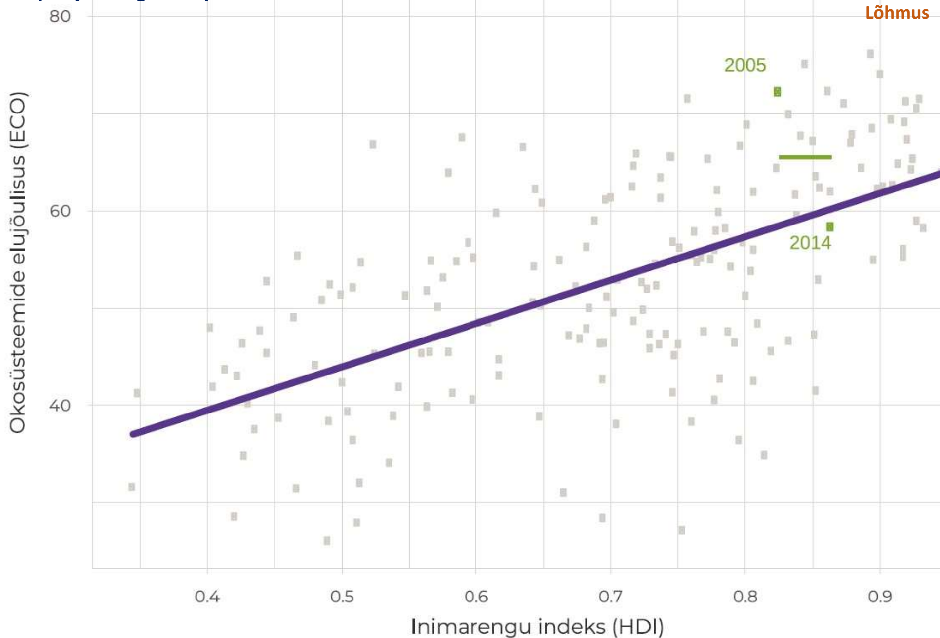
Joonis 3.0.1. Inimarengu indeksi ja ökosüsteemide elujõulisuse indeksi seos 179 riigi põhjal ning Eesti positsiooni muutus 2005–2014
